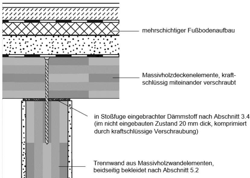
Prinzipskizze 8c: Anschluss Trennwand / Massivholzdecke, Bauteilfuge (Vertikalschnitt)
