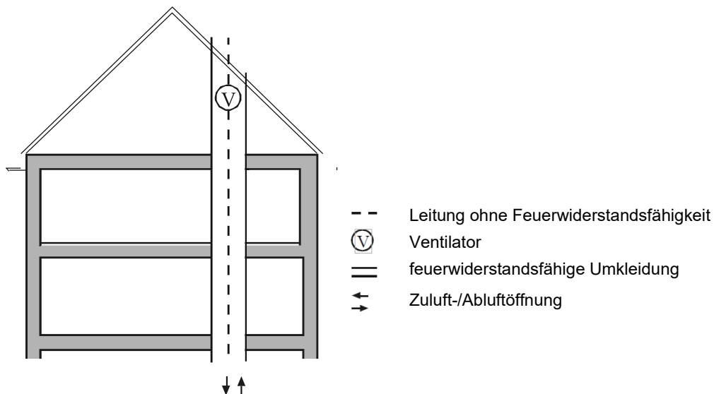
Bild 2.2: Schachtlösung
