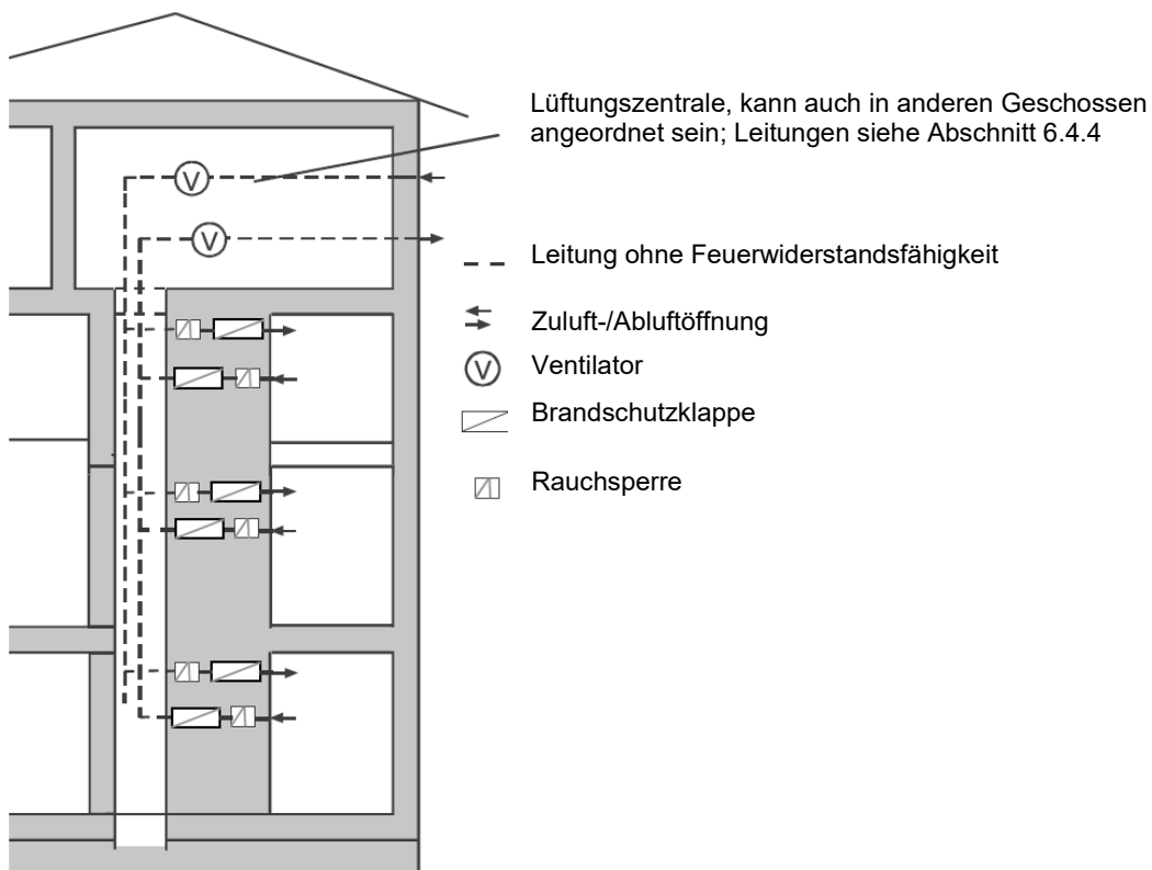
Bild 6.1: Lüftungsanlagen zur Be- und Entlüftung von Wohnungen bzw. abgeschlossene Nutzungseinheiten max. 200 m 2
