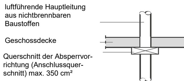
Bild 6.2: Beispiel für Schottlösung für Lüftungsanlagen nach DIN 18017 3:2022-05 maximaler Anschlussquerschnitt der Absperrvorrichtungen: 350 cm 2
