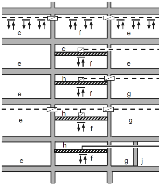
Bild 3.2: notwendiger Flur belüftet
