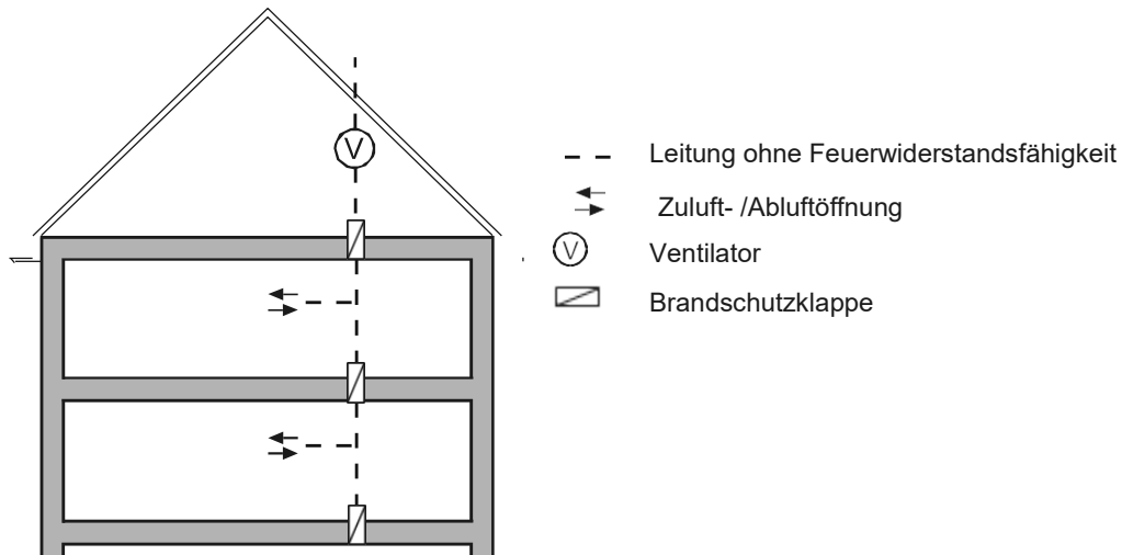
Bild 2.1: Schottlösung
