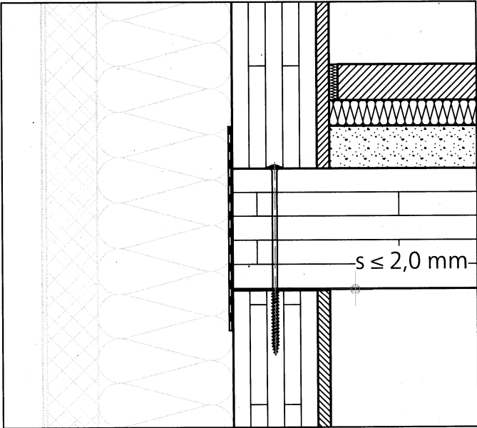
Abbildung 15: Außenwand-Deckenanschlüsse Massivholzbau mit Spaltmaß s \leq 2,0 \text{ mm}
