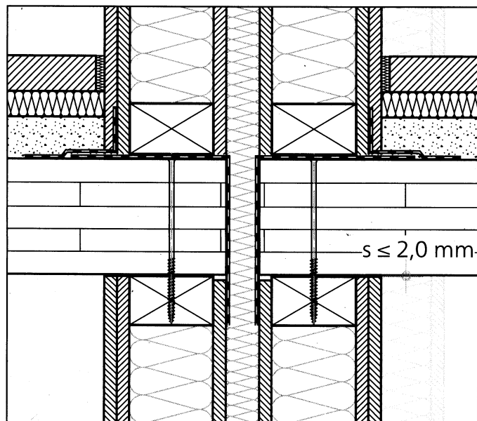
Abbildung 30: Trennwand-Deckenanschlüsse Holztafelbau / Massivholzbau mit Spaltmaß s \leq 2,0 mm
