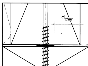
Abbildung 8: Trennwand-Deckenanschlüsse Holztafelbau mit Spaltmaß s \leq 2,0 mm
