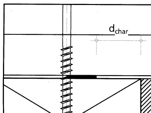
Abbildung 30: Trennwand-Deckenanschlüsse Holztafelbau / Massivholzbau mit Spaltmaß s \leq 2,0 mm
