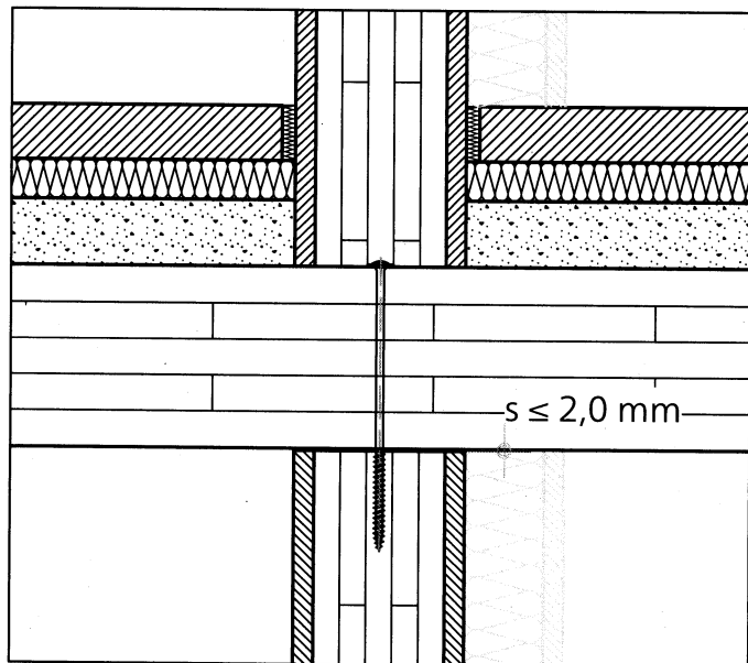
Abbildung 16: Trennwand-Deckenanschlüsse Massivholzbau mit Spaltmaß s \leq 2,0 mm
