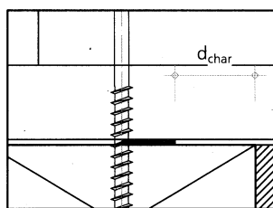
Abbildung 29: Trennwand-Deckenanschlüsse Holztafelbau / Massivholzbau mit Spaltmaß s \leq 2,0 \text{ mm}
