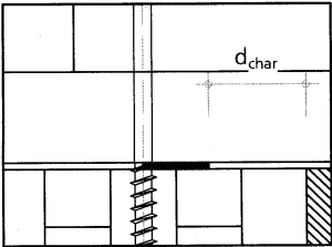
Abbildung 15: Außenwand-Deckenanschlüsse Massivholzbau mit Spaltmaß s \leq 2,0 \text{ mm}
