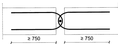
Bild: Vertikale Stoßfuge in Wandebene bei Brandwänden
