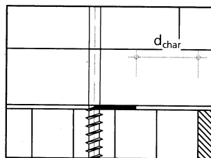
Abbildung 16: Trennwand-Deckenanschlüsse Massivholzbau mit Spaltmaß s \leq 2,0 mm
