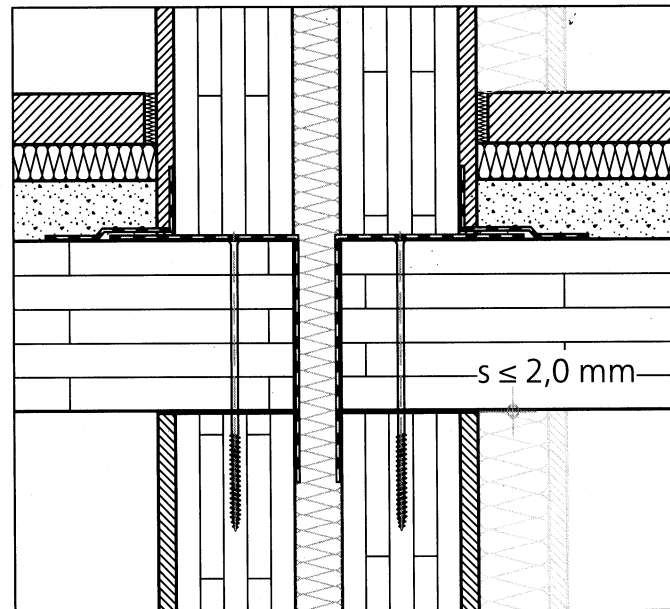
Abbildung 19: Trennwand-Deckenanschluss Massivholzbau mit Spaltmaß s \leq 2,0 mm
