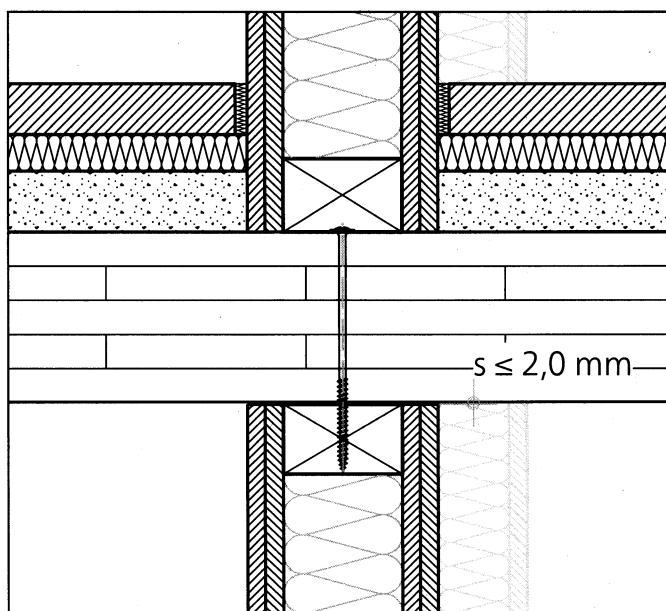
Abbildung 29: Trennwand-Deckenanschlüsse Holztafelbau / Massivholzbau mit Spaltmaß s \leq 2,0 \text{ mm}
