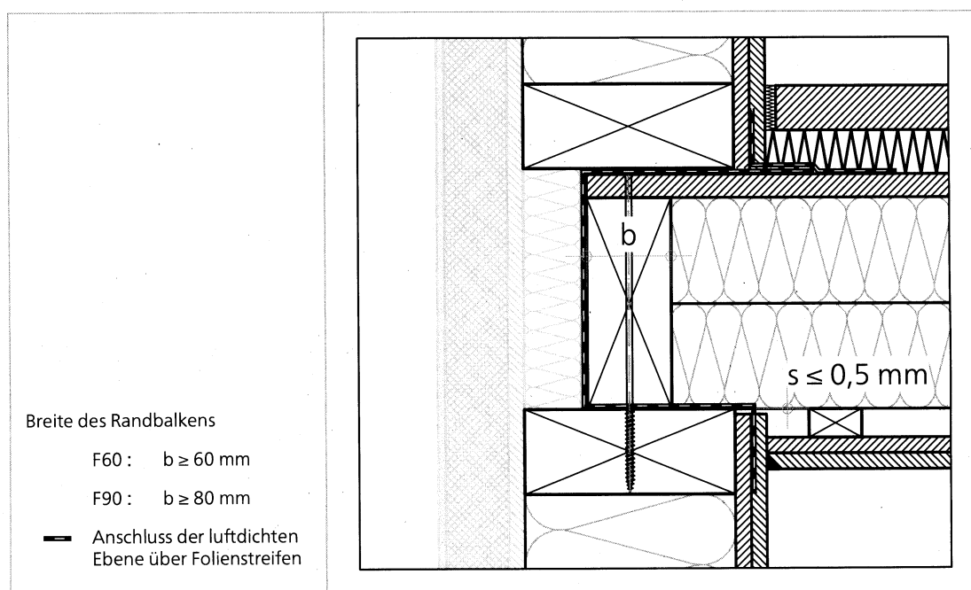
Abbildung 5: Außenwand-Deckenanschluss Holztafelbau mit Spaltmaß s \leq 0,5 \text{ mm}
