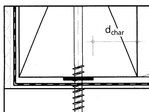
Abbildung 7: Außenwand-Deckenanschlüsse Holztafelbau mit Spaltmaß s \leq 2,0 \text{ mm}
