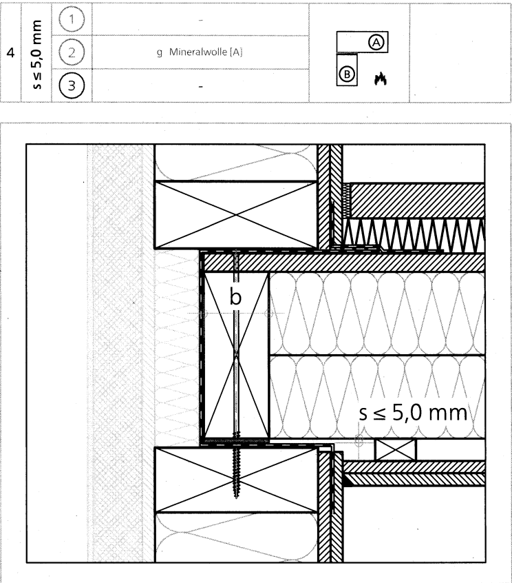
Abbildung 11: Außenwand-Deckenanschluss Holztafelbau mit Spaltmaß s ≤ 5,0 mm
