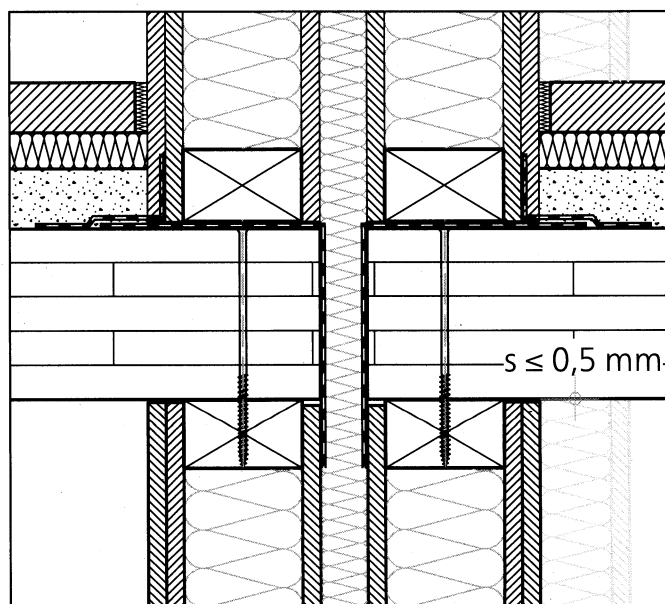
Abbildung 27: Trennwand-Deckenanschlüsse Holztafelbau / Massivholzbau mit Spaltmaß s \leq 0,5 mm
