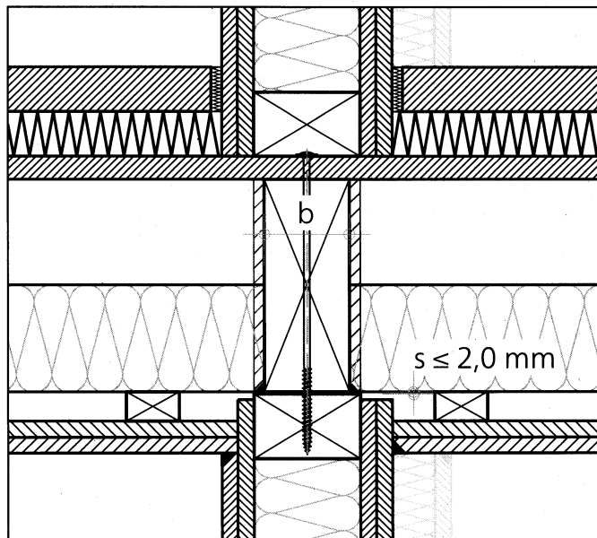
Abbildung 9: Trennwand-Deckenanschluss Holztafelbau mit Spaltmaß s \leq 2,0 mm
