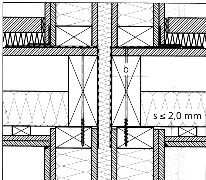
Abbildung 10: Trennwand-Deckenanschlüsse Holztafelbau mit Spaltmaß s \leq 2,0 \text{ mm}
