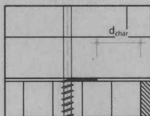
Abbildung 16: Trennwand-Deckenanschlüsse Massivholzbau mit Spaltmaß s \leq 2,0 mm
