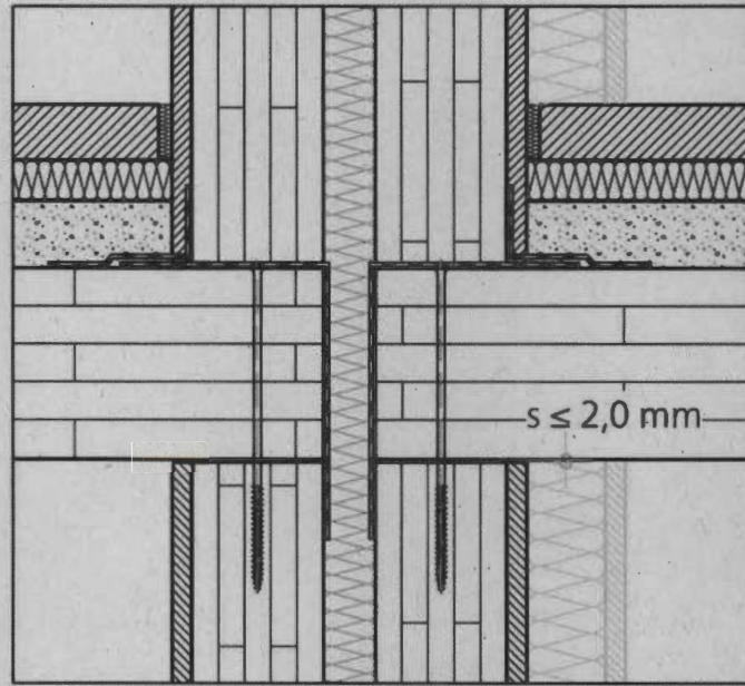
Abbildung 19: Trennwand-Deckenanschluss Massivholzbau mit Spaltmaß s \leq 2,0 \text{ mm}
