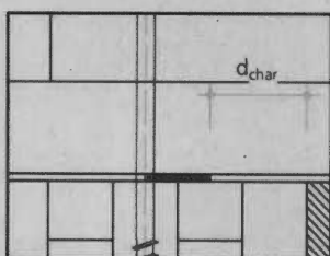
Abbildung 17: Trennwand-Deckenanschlüsse Massivholzbau mit Spaltmaß s \leq 2,0 mm
