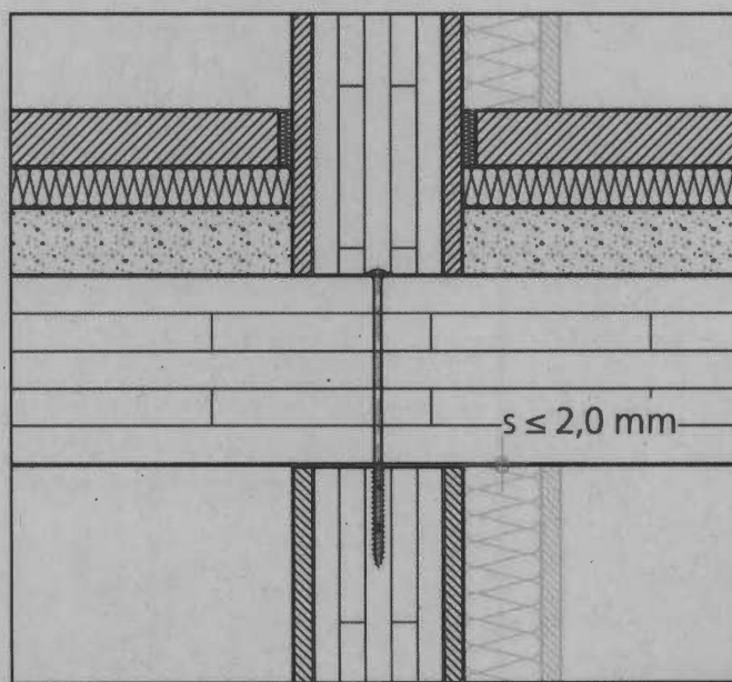
Abbildung 16: Trennwand-Deckenanschlüsse Massivholzbau mit Spaltmaß s \leq 2,0 mm
