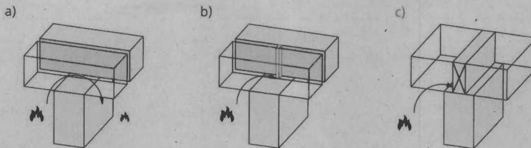
Abbildung 4: Brandübertragungspfade durch flankierende Bauteile: a) Brandübertragung über ein raumabschließendes Bauteil hinweg über durchgehende Elementfugen, b) Dichtungsmaßnahme in den Elementfugen, c) Verblockung innerhalb des Bauteils
