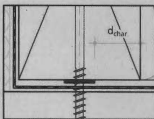
Abbildung 7: Außenwand-Deckenanschlüsse Holztafelbau mit Spaltmaß s \leq 2,0 mm
