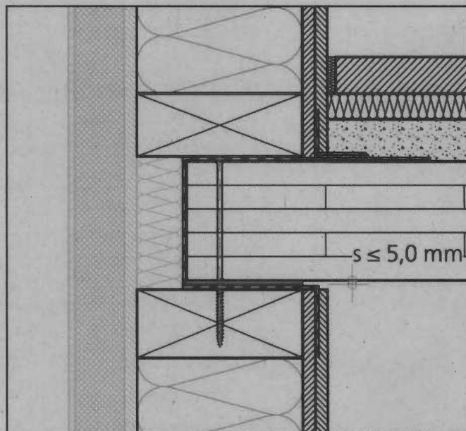
Abbildung 32: Außenwand-Deckenanschluss Holztafelbau / Massivholzbau mit Spaltmaß s \leq 5,0\text{ mm}
