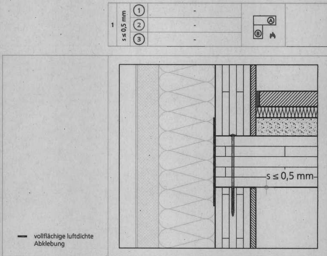
Abbildung 13: Außenwand-Deckenanschluss Massivholzbau mit Spaltmaß s \leq 0,5 \text{ mm}
