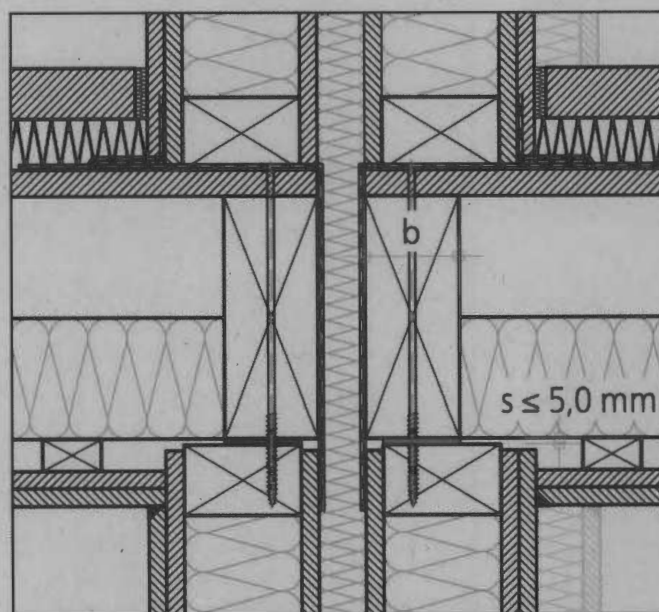
Abbildung 12: Trennwand-Deckenanschlüsse Holztafelbau mit Spaltmaß s \leq 5,0 \text{ mm}
