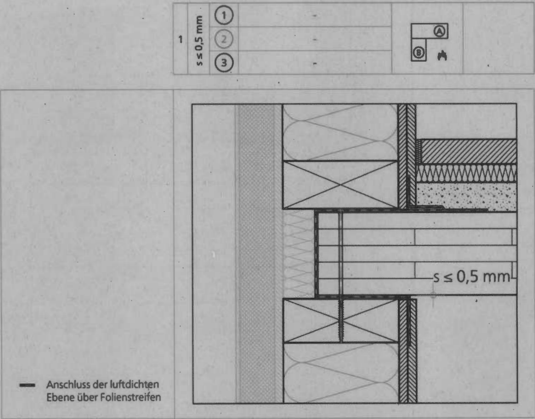
Abbildung 26: Außenwand-Deckenanschluss Holztafelbau / Massivholzbau mit Spaltmaß s \leq 0,5 \text{ mm}
