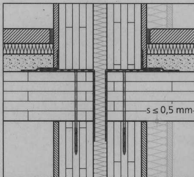
Abbildung 14: Trennwand-Deckenanschlüsse Massivholzbau mit Spaltmaß s \leq 0,5 mm
