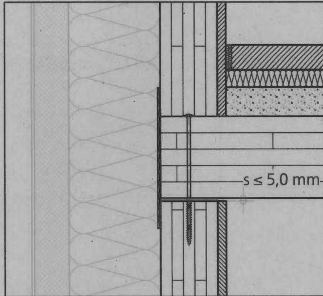
Abbildung 20: Außenwand-Deckenanschluss Massivholzbau mit Spaltmaß s \leq 5,0 \text{ mm}
