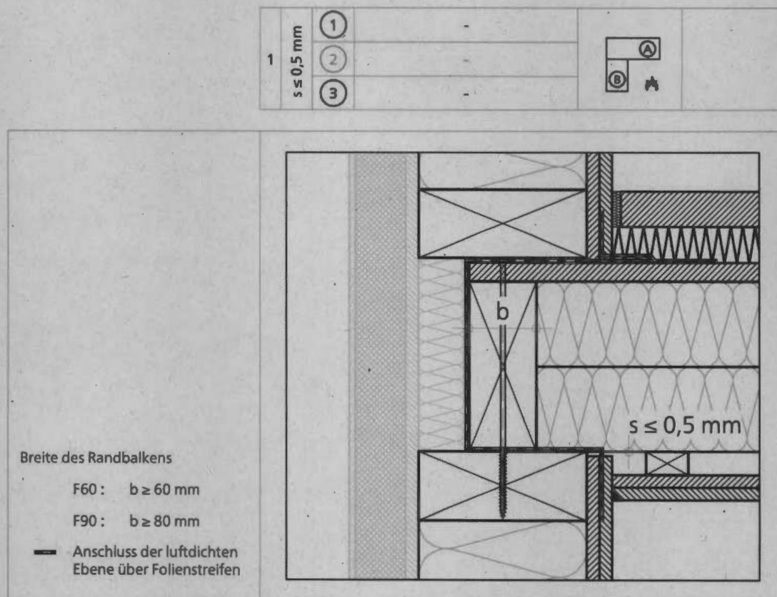
Abbildung 5: Außenwand-Deckenanschluss Holztafelbau mit Spaltmaß s \leq 0,5 \text{ mm}
