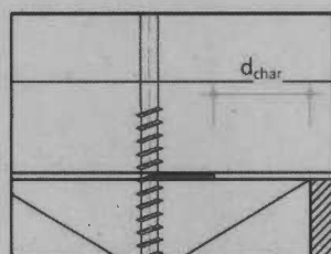
Abbildung 30: Trennwand-Deckenanschlüsse Holztafelbau / Massivholzbau mit Spaltmaß s \leq 2,0 \text{ mm}
