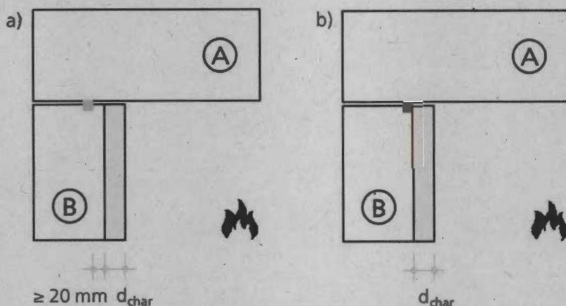
Abbildung 3: Position einer dauerelastischen Abdichtung im Bauteil: a) Ausführung mit dauerelastischer Verfugung / Dichtstoff; b) Ausführung mit Brandschutzdichtmasse; d_{\text{char}} nach DIN 1995-1-2
