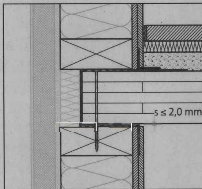
Abbildung 28: Außenwand-Deckenanschlüsse Holztafelbau / Massivholzbau mit Spaltmaß s \leq 2,0 mm
